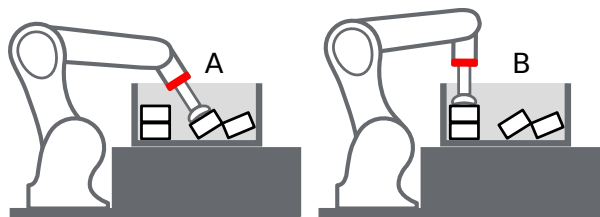
Abb. 5.42: Fall A: Der Griff wird nur als Kollision erkannt, wenn check_flange auf true gesetzt ist, denn der Flansch (rot) befindet sich im Load Carrier. Fall B: Der Griff ist in jedem Fall kollisionsfrei.
