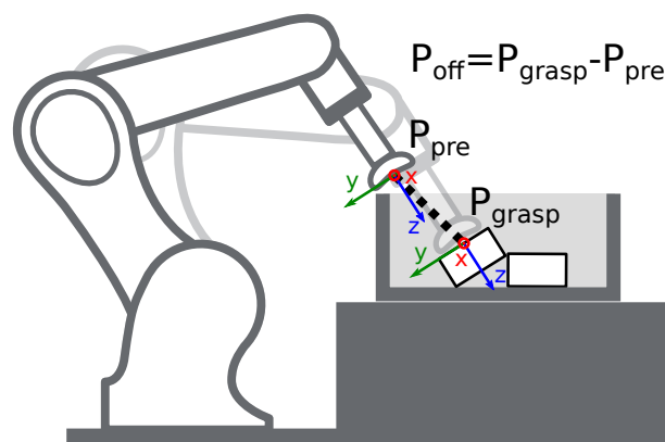
Abb. 6.27: Darstellung des Greif-Offsets für die Kollisionsprüfung. Im dargestellten Fall sind sowohl die Vorgreifposition als auch die Greifposition kollisionsfrei, aber die Trajektorie zwischen diesen Punkten hätte eine Kollision mit dem Load Carrier. Deswegen wird dieser Greifpunkt als Kollision erkannt.
