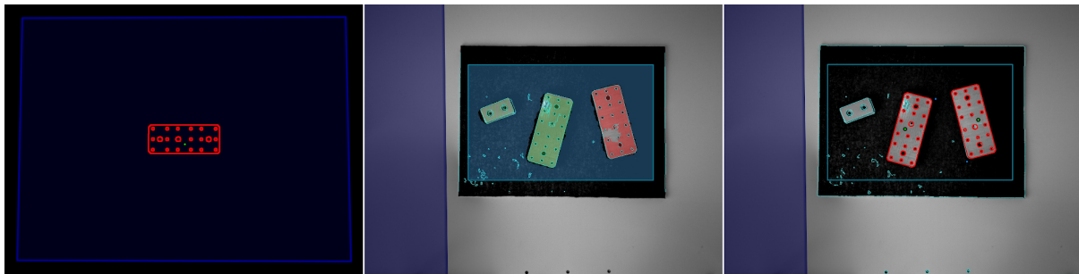
Abb. 6.16: „Template“, „Zwischenergebnis“ und „Ergebnis“ Bilder des SilhouetteMatch Moduls in der Web GUI für eine Detektion mit automatischer Objektebenenerkennung ( object_plane_detection ist true)
