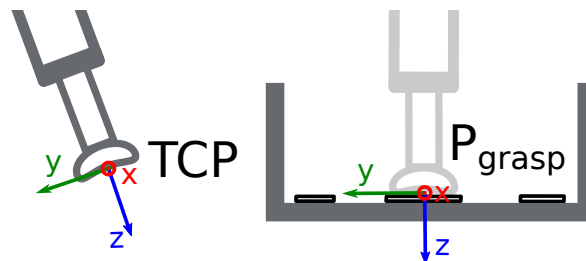
Abb. 6.15: Definition von Greifpunkten bezogen auf den Roboter-TCP
