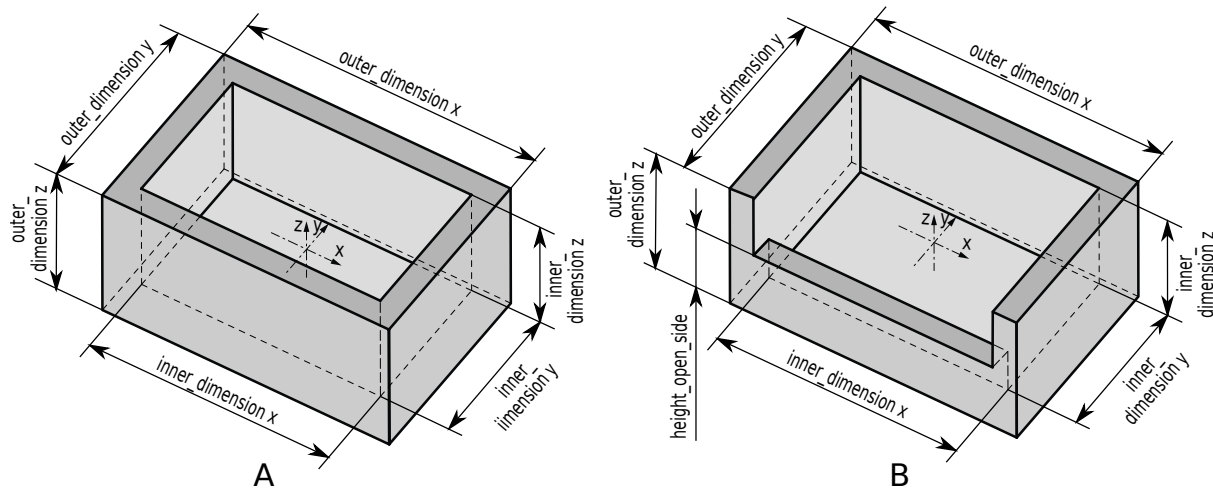
Abb. 6.41: Beispiele eines 4-seitigen (A) und 3-seitigen Load Carriers (B)
