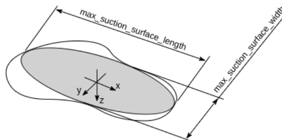
Abb. 6.12: Veranschaulichung eines berechneten Greifpunktes mit Koordinatensystem und der zugehörigen Ellipse, welche die Greiffläche bestmöglich beschreibt.
