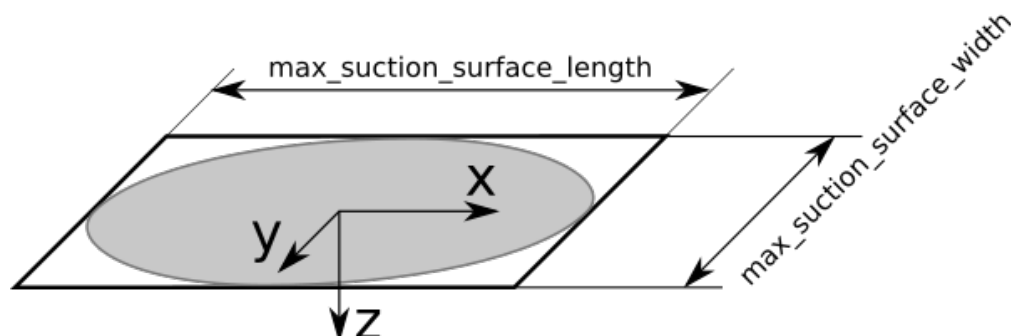
Abb. 6.13: Veranschaulichung eines berechneten Greifpunktes mit Koordinatensystem und der zugehörigen Ellipse, welche die größtmögliche Greiffläche beschreibt.
