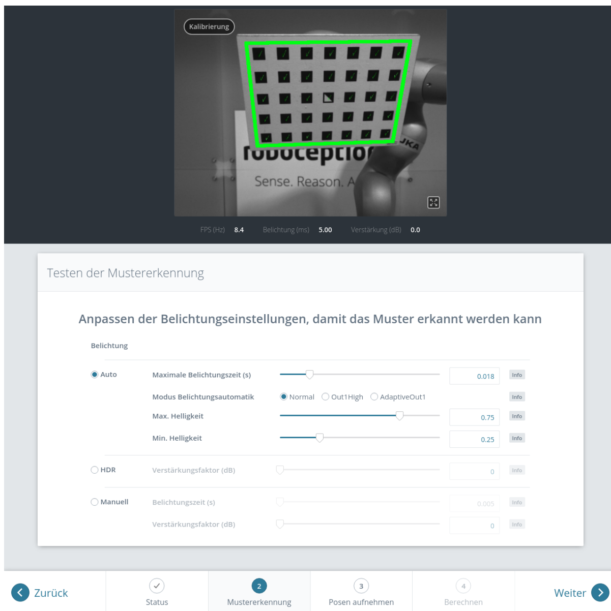
Abb. 6.23: Testen der Mustererkennung
