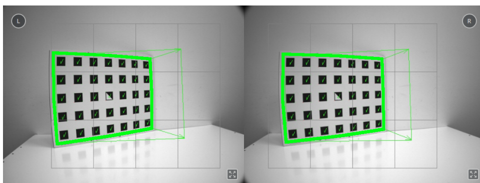
Abb. 6.31: Pfeile weisen darauf hin, wenn das Muster während der Stereokalibrierung nicht senkrecht zur Blickrichtung der Kamera gehalten wird.
