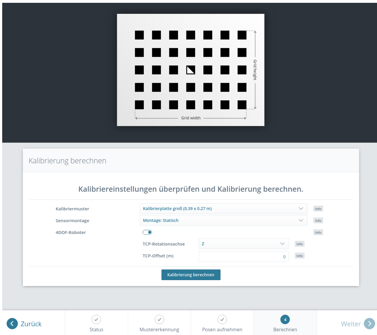
Abb. 6.26: Setzen der Parameter und Berechnen der Hand-Auge-Kalibrierung in der Web GUI des rc_cube
