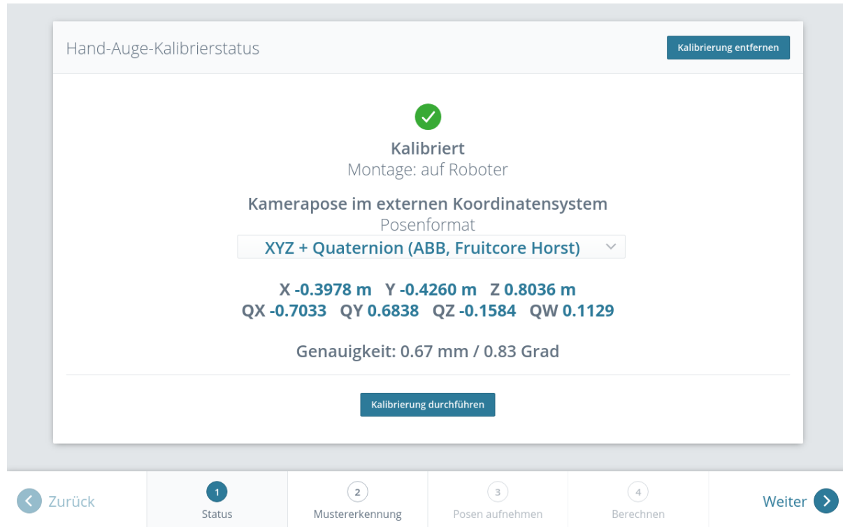
Abb. 6.22: Aktueller Status der Hand-Auge-Kalibrierung falls eine Hand-Auge-Kalibrierung gespeichert ist
