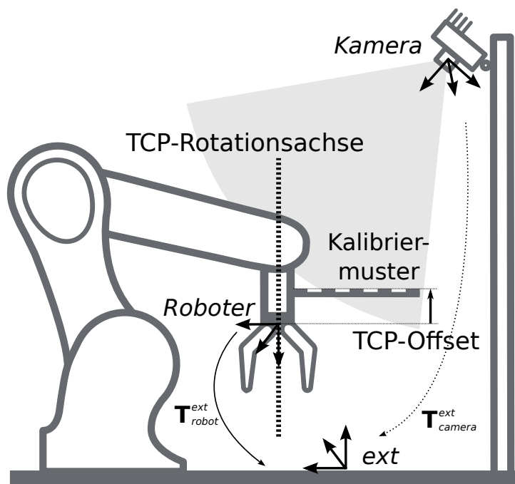
Abb. 6.20: Im Fall eines 4DOF-Roboters müssen die TCP-Rotationsachse und der Offset vom TCP zur sichtbaren Oberfläche des Kalibrierusters entlang der TCP-Rotationsachse angegeben werden. Im dargestellten Fall ist der Offset negativ.
