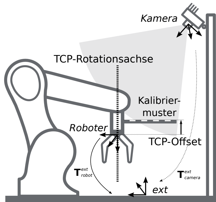
Abb. 6.20: Im Fall eines 4DOF-Roboters müssen die TCP-Rotationsachse und der Offset vom TCP zur sichtbaren Oberfläche des Kalibrieremusters entlang der TCP-Rotationsachse angegeben werden. Im dargestellten Fall ist der Offset negativ.
