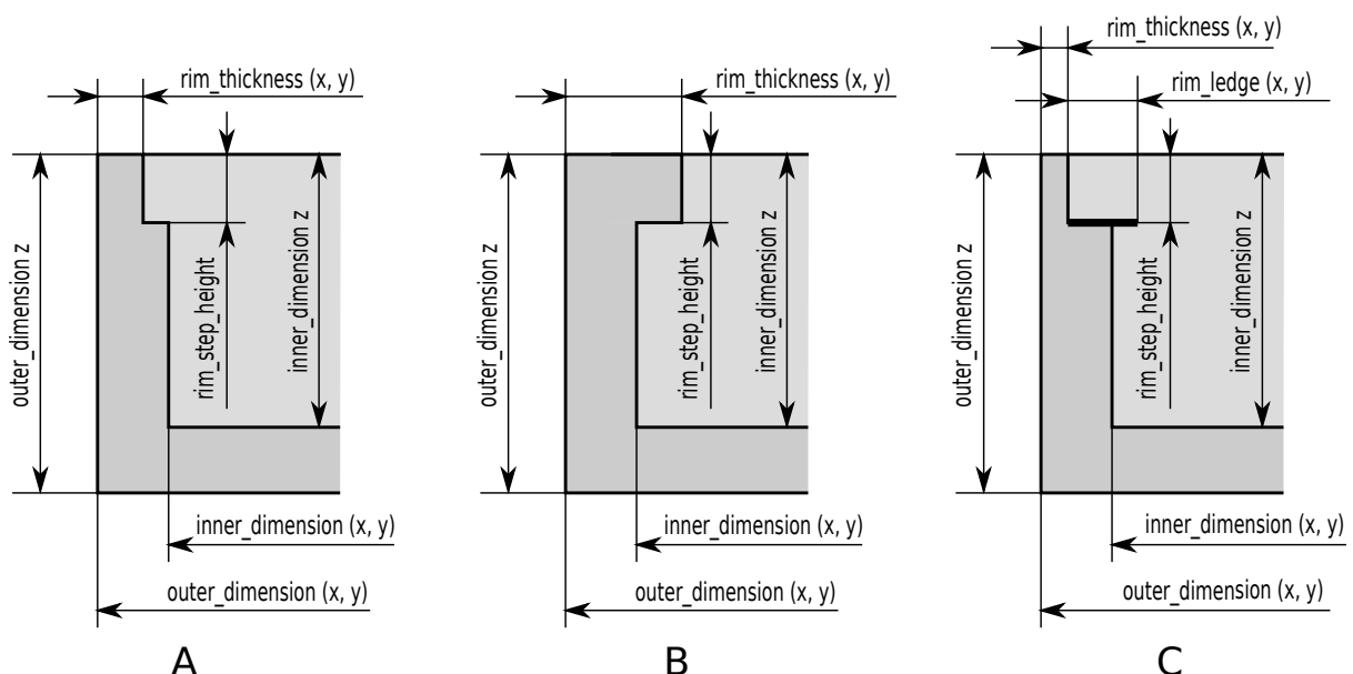
Abb. 6.40: Beispiele von Load Carriern mit abgestuften (A, B) und vorspringendem Rand (C)
