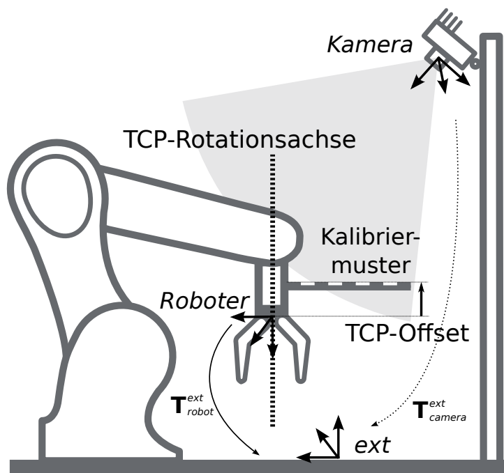
Abb. 5.23: Im Fall eines 4DOF-Roboters müssen die TCP-Rotationsachse und der Offset vom TCP zur sichtbaren Oberfläche des Kalibrieremusters entlang der TCP-Rotationsachse angegeben werden. Im dargestellten Fall ist der Offset negativ.
