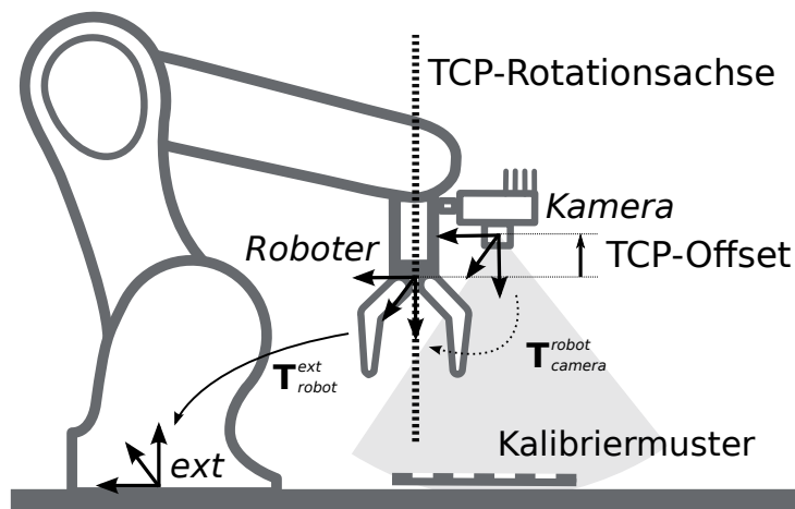
Abb. 5.20: Im Fall eines 4DOF-Roboters müssen die TCP-Rotationsachse und der Offset vom TCP zum Kamerakoordinatensystem entlang der TCP-Rotationsachse angegeben werden. Im dargestellten Fall ist der Offset negativ.
