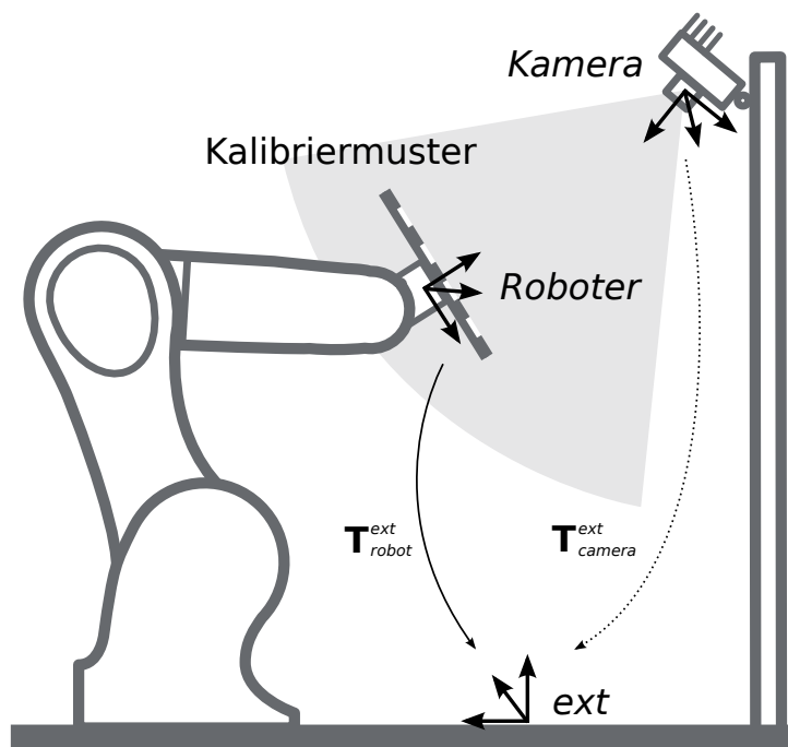
Abb. 5.21: Wichtige Koordinatensysteme und Transformationen für die Kalibrierung einer statisch montierten Kamera: Sie wird mit einer festen Position relativ zu einem benutzerdefinierten externen Referenzkoordinatensystem ext (z.B. Weltkoordinatensystem oder Roboter-Montagepunkt) montiert. Es ist wichtig, dass die Pose T_{robot}^{ext} des benutzerdefinierten Roboter -Koordinatensystems in Bezug auf dieses Koordinatensystem während der Kalibrierroutine gemessen werden kann. Das Ergebnis des Kalibrierprozesses ist die gewünschte Kalibriertransformation T_{camera}^{ext} , d.h. die Pose des Kamera -Koordinatensystems im benutzerdefinierten externen Koordinatensystem ext .
