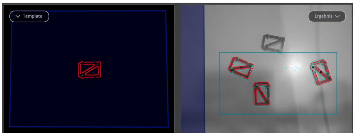
Abb. 5.17: Ergebnisbild des SilhouetteMatch-Moduls, wie über die Web GUI dargestellt
