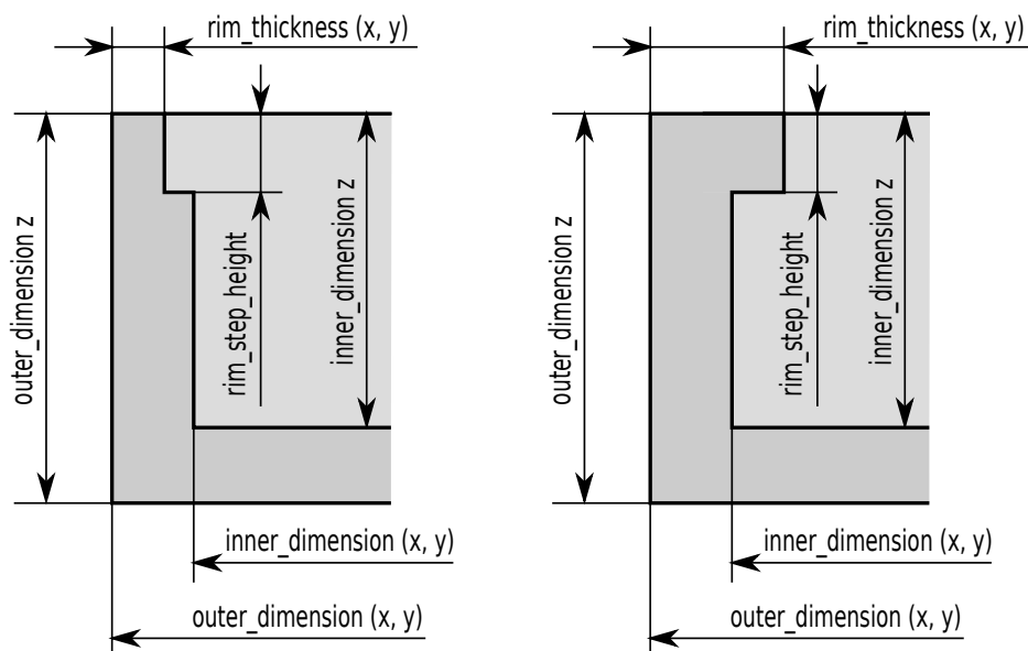
Abb. 5.6: Beispiele für Load Carrier, bei denen die Angabe der Randstärke für die Erkennung notwendig ist
