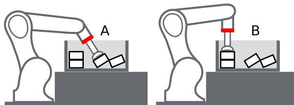
Abb. 5.30: Fall A: Der Griff wird nur als Kollision erkannt, wenn check_flange auf true gesetzt ist, denn der Flansch (rot) befindet sich im Load Carrier. Fall B: Der Griff ist in jedem Fall kollisionsfrei.
