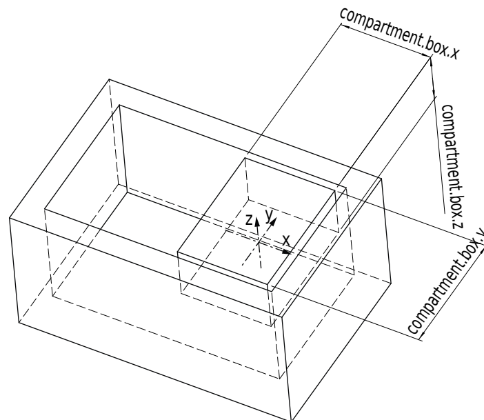
Abb. 5.7: Beispiel für ein Abteil innerhalb eines Load Carriers. Das gezeigte Koordinatensystem des Load Carrier Abteils.
