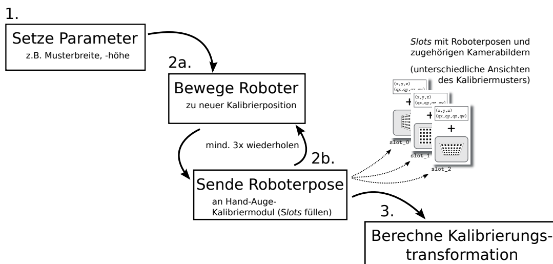
Abb. 5.24: Darstellung der drei Schritte der Hand-Auge-Kalibrierroutine
