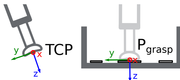
Abb. 5.16: Definition von Greifpunkten bezogen auf den Roboter-TCP
