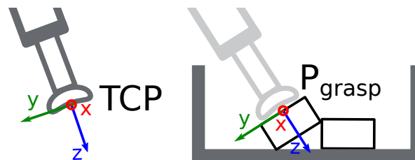
Abb. 5.18: Definition von Greifpunkten bezogen auf den Roboter-TCP
