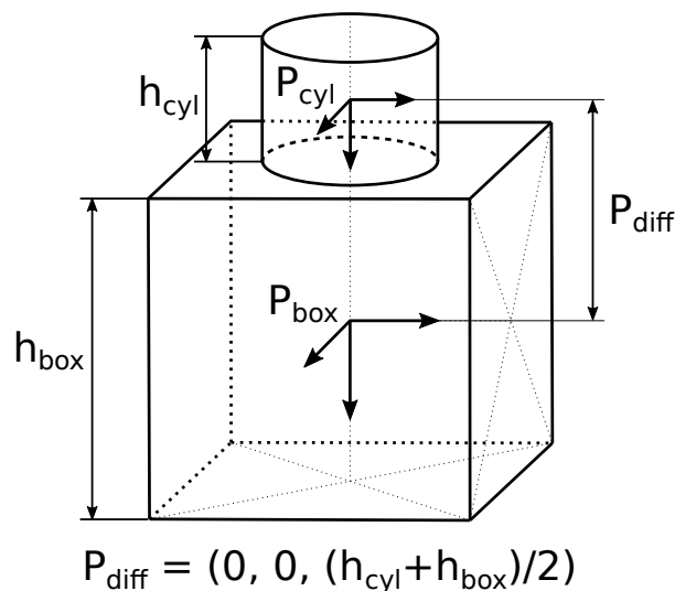
Abb. 5.31: Bezugskoordinatensysteme für das Erstellen von Greifern über die REST-API
