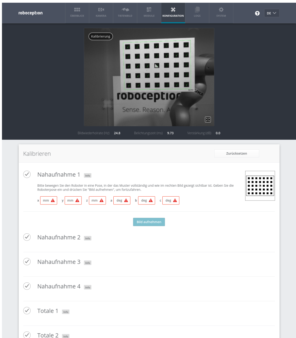
Abb. 5.27: Erstes Beispielbild für den Hand-Auge-Kalibriervorgang einer statisch montierten Kamera
