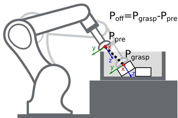
Abb. 5.32: Darstellung des Greif-Offsets für die Kollisionsprüfung. Im dargestellten Fall sind sowohl die Vorgreifposition als auch die Greifposition kollisionsfrei, aber die Trajektorie zwischen diesen Punkten hätte eine Kollision mit dem Load Carrier. Deswegen wird dieser Greifpunkt als Kollision erkannt.
