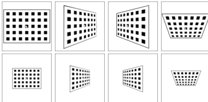
Abb. 5.26: Empfohlene Ansichten des Kalibrierusters während des Kalibriervorgangs. Im Fall von 4DOF-Robotern müssen andere Ansichten gewählt werden, welche so unterschiedlich wie möglich sein sollten.
