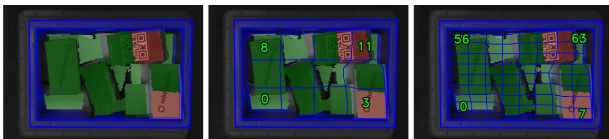
Abb. 5.9: Visualisierungen des Behälterfüllstands: Gesamtfüllstand ohne Raster (links), 4x3 Raster (Mitte), 8x8 Raster (rechts). Der Inhalt wird mit einem Farbverlauf von weiß (auf dem Boden) nach dunkelgrün dargestellt. Die überfüllten Bereiche sind rot dargestellt. Die Nummern stellen die Zell-IDs dar.
