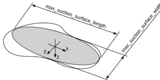
Abb. 5.15: Veranschaulichung eines berechneten Greifpunktes mit Greifpose und der zugehörigen Ellipse, welche die Greiffläche bestmöglich beschreibt.
