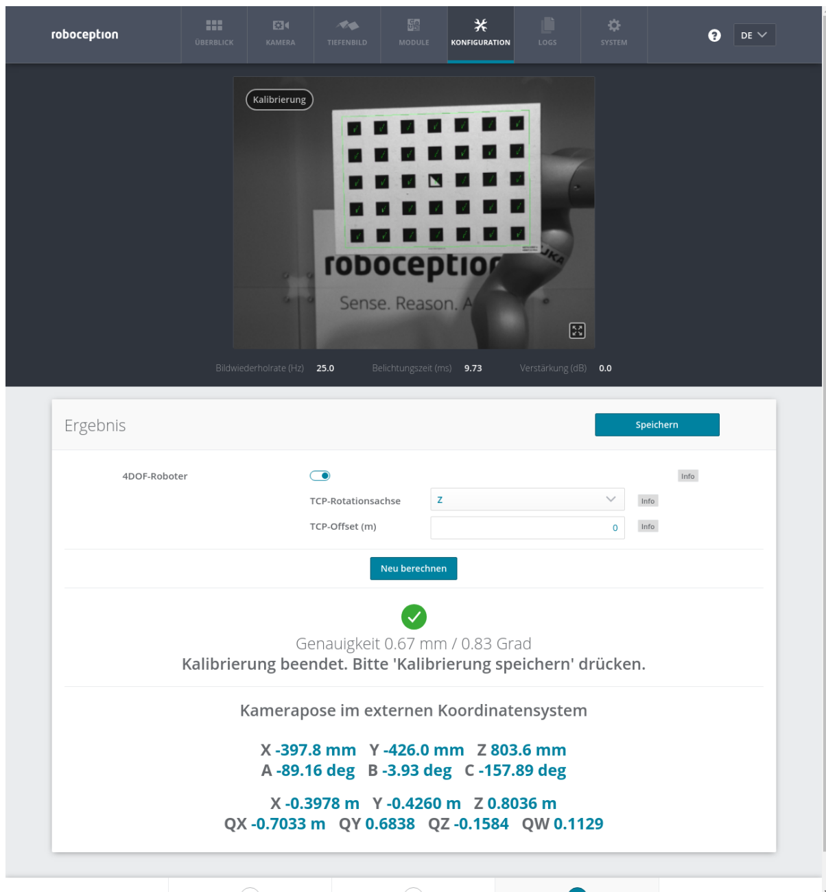
Abb. 5.29: Ergebnis der Hand-Auge-Kalibrierung, dargestellt in der Web GUI
