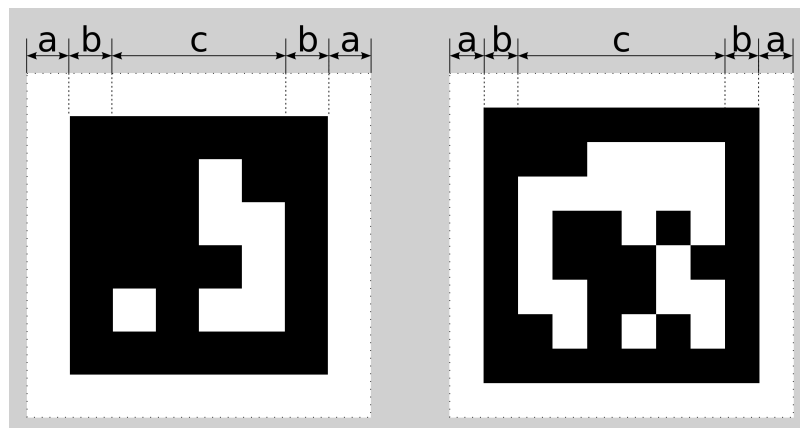
Abb. 5.11: Ein 16h5 Marker (links) und ein 36h11 Marker (rechts). AprilTags bestehen aus einem obligatorischen weißen (a) und schwarzen (b) Rahmen und einer variablen Menge an Datenmodulen (c).
