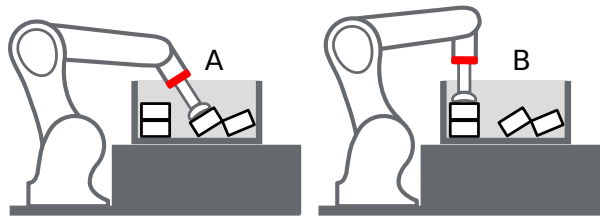
Abb. 5.30: Fall A: Der Griff wird nur als Kollision erkannt, wenn check_flange auf true gesetzt ist, denn der Flansch (rot) befindet sich im Load Carrier. Fall B: Der Griff ist in jedem Fall kollisionsfrei.
