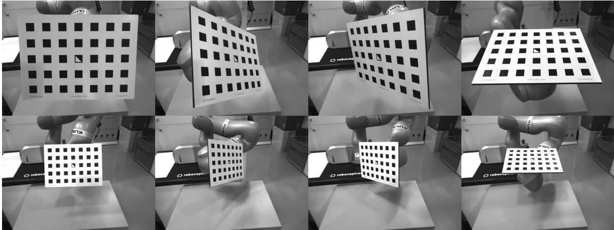
Abb. 5.28: Beispiel-Kamerabilder für die Hand-Auge-Kalibrierung
