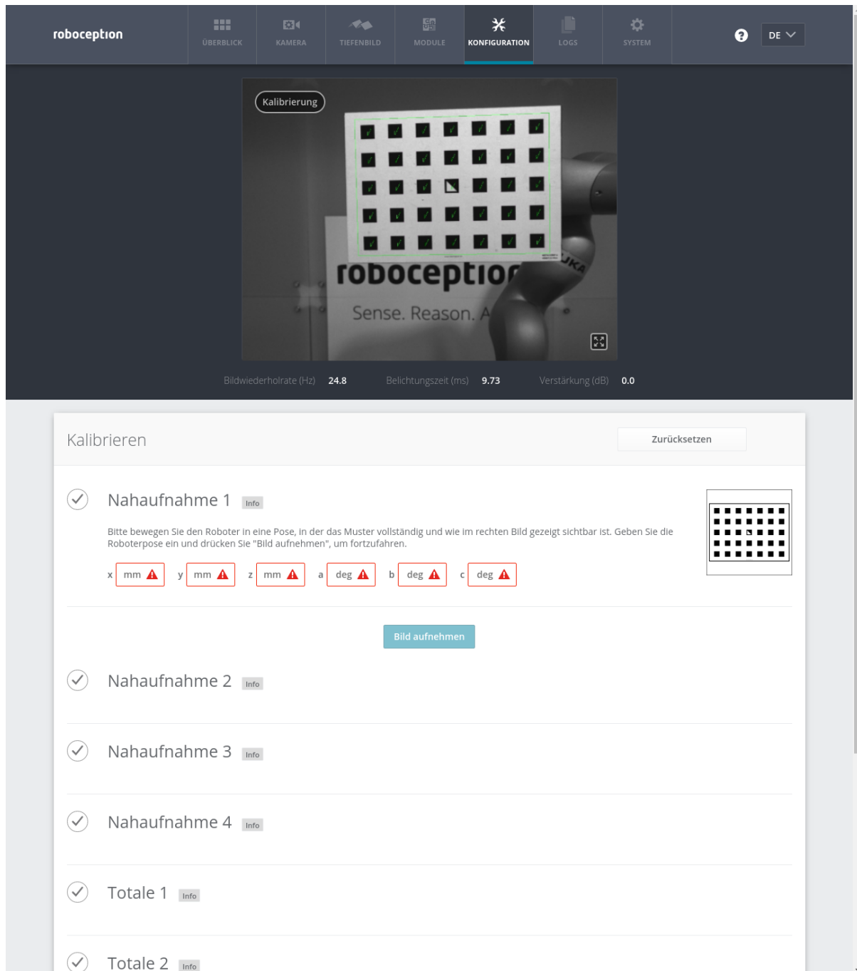
Abb. 5.27: Erstes Beispielbild für den Hand-Auge-Kalibriervorgang einer statisch montierten Kamera
