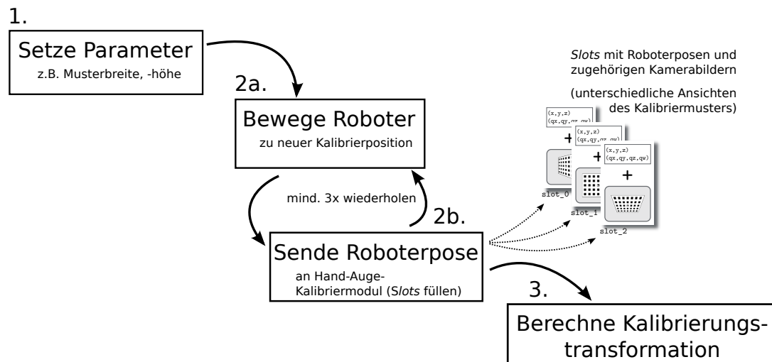
Abb. 5.24: Darstellung der drei Schritte der Hand-Auge-Kalibrieroutine
