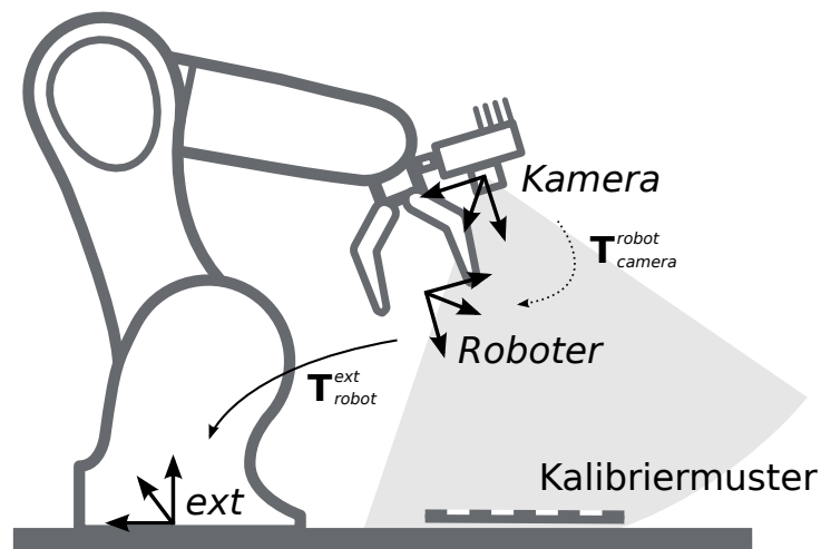
Abb. 5.19: Wichtige Koordinatensysteme und Transformationen für die Kalibrierung einer robotergeführten Kamera: Sie wird mit einer festen relativen Position zu einem benutzerdefinierten Roboter -Koordinatensystem (z.B. Flansch oder Werkzeugmittelpunkt) montiert. Es ist wichtig, dass die Pose T_{robot}^{ext} des Roboter -Koordinatensystems in Bezug auf ein benutzerdefiniertes externes Referenzkoordinatensystem ( ext ) während der Kalibrierroutine gemessen werden kann. Das Ergebnis des Kalibriervorgangs ist die gewünschte Kalibriertransformation T_{camera}^{robot} , d.h. die Pose des Kamera -Koordinatensystems im benutzerdefinierten Roboter -Koordinatensystem.
