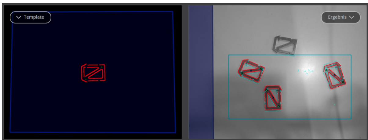
Abb. 5.17: Ergebnisbild des SilhouetteMatch-Moduls, wie über die Web GUI dargestellt
