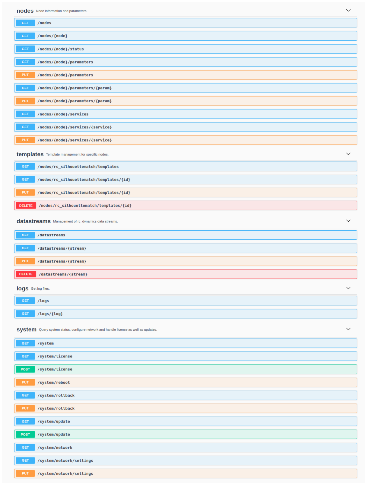
Abb. 6.2: Startansicht der Swagger UI des rc_cube , bei der die Ressourcen und Anfragen in nodes, templates, datastreams, logs und system gruppiert sind.
