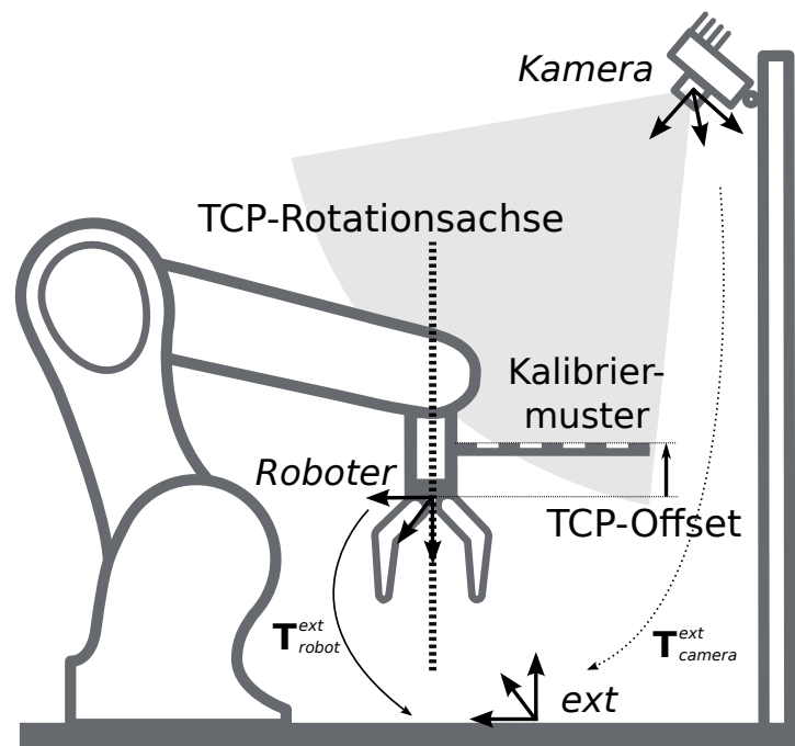
Abb. 5.23: Im Fall eines 4DOF-Roboters müssen die TCP-Rotationsachse und der Offset vom TCP zur sichtbaren Oberfläche des Kalibrieramusters entlang der TCP-Rotationsachse angegeben werden. Im dargestellten Fall ist der Offset negativ.
